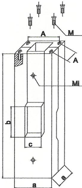
Fundament prefabrykowany Typ FB-W150
