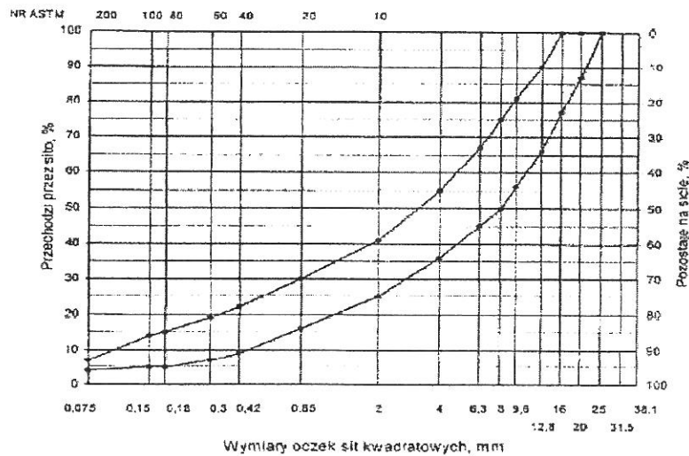
Rys. 2. Krzywe graniczne uziarnienia mieszanki mineralnej BA od 0 do 20 mm do warstwy wiążącej nawierzchni drogi o obciążeniu ruchem od KR3
